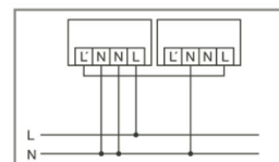
Standardbetrieb mit zusätzlichem Anschluss von externen Lasten.
